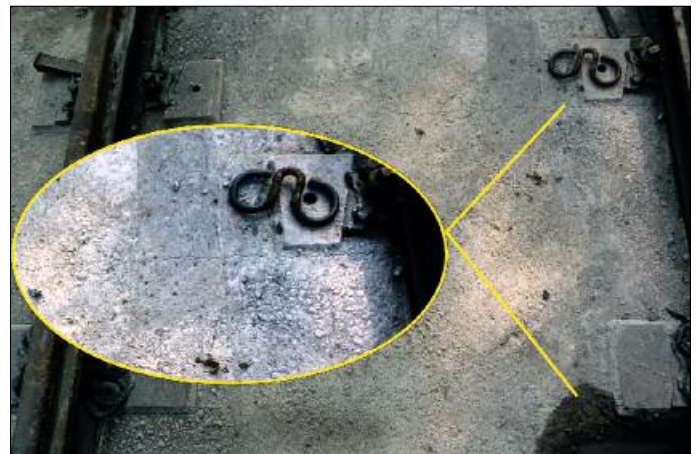
4. Typisches Rissbild in der Tragkonstruktion
