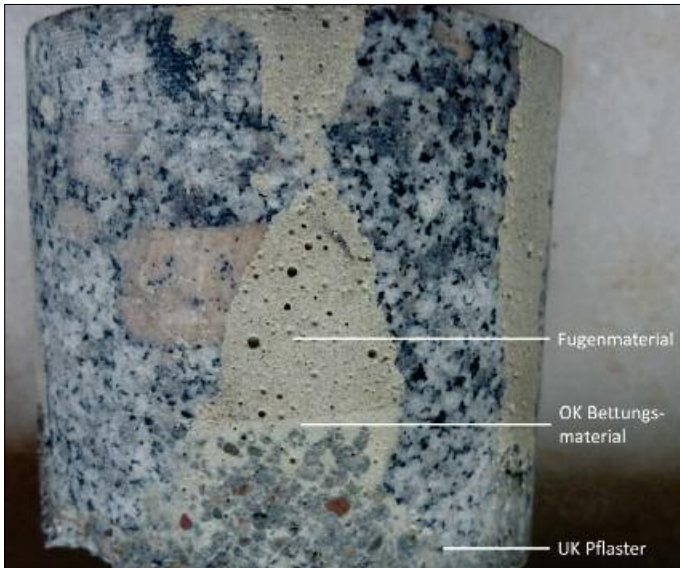
6. Beispiel für die Ausführbarkeit von Bettungskleberschicht und Verfugung Abbildung: DVB
