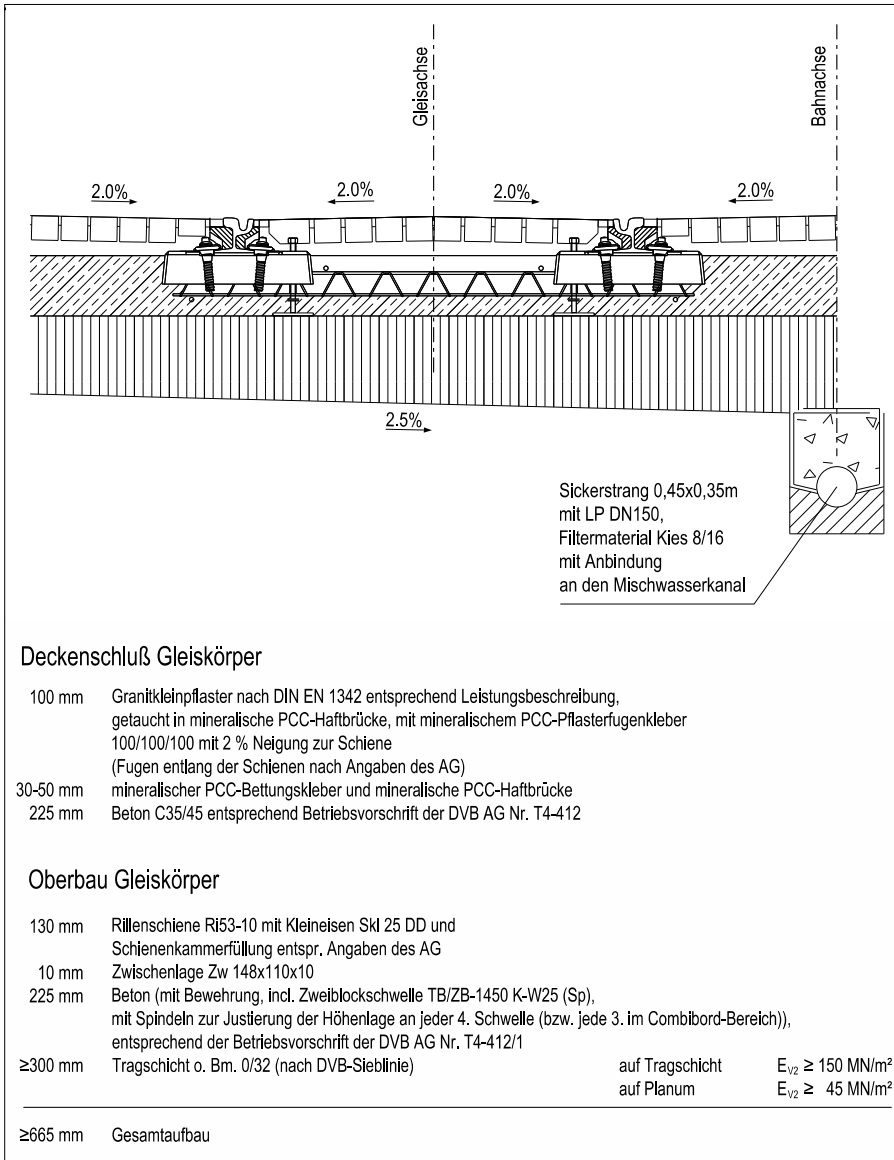
2. Regelquerschnitt eines Gleises in monolithischer Pflasterbauweise mit Schienenprofil Ri 53-10, vgl. [4] Abbildung: DVB
