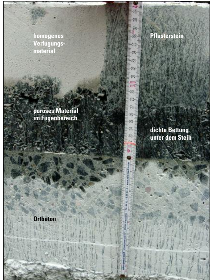
7. Querschnitt durch den vollgebundenen Oberbau (Naturstein, Verfugung, Bettungsschicht, Betontragschicht) Abbildung: K. Jordan
